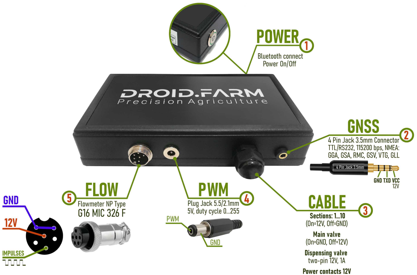
Рис. 2. Внешний вид SC10 (не в масштабе 1:1)
